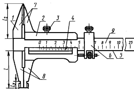
1 — штанга; 2 — рамка; 3 — зажимающий элемент; 4 — нониус; 5 — рабочая поверхность штанги; 6 — устройство тонкой установки рамки; 7 — губки с кромочными измерительными поверхностями для измерения наружных размеров; 8 — губки с плоскими измерительными поверхностями для измерения наружных и внутренних размеров соответственно; 9 — шкала штанги Largest alloy pipe, fitting, flange supplier www.cnpipefitting.com Email: alloypipefitting@gmail.com
