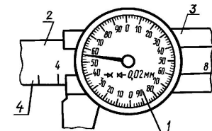
1 — круговая шкала отсчетного устройства; 2 — штанга; 3 — рамка; 4 — шкала штанги
